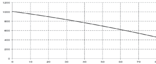
*Καμπύλη Απόδοσης του συλλέκτη 2NLO 25 σε ηλιακή ακτινοβολία 1000W/m 2 (Πιστοποιημένος με Solar Keymark)
