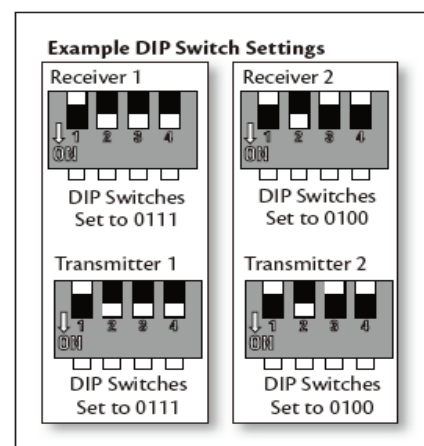
Fig. 11 DIP-schakelaar ontvanger
